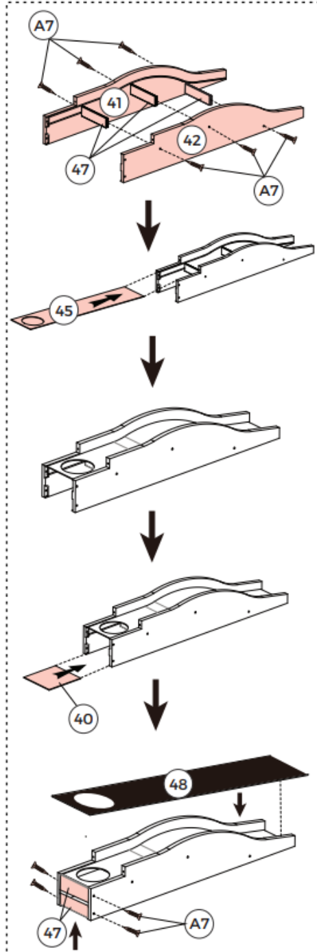
FIG. 10A Assembly
